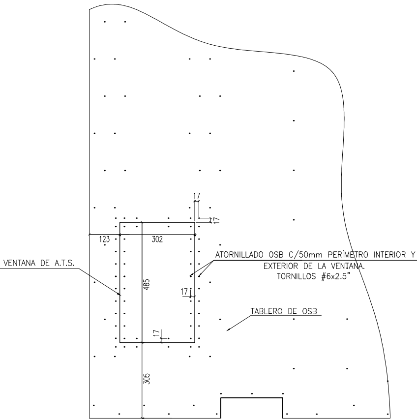
DETALLE DE FIJACIÓN DE OSB EN VENTANA DE ATS
