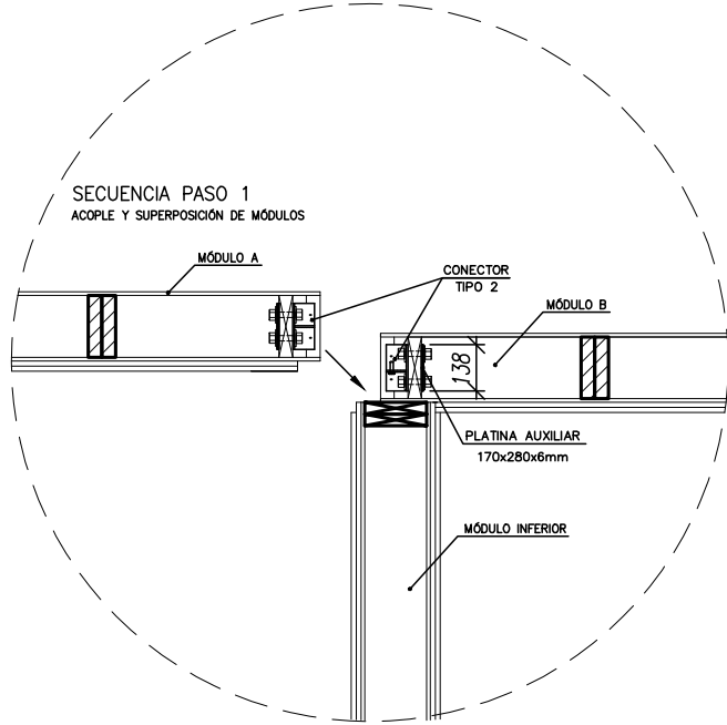
Detalle Conexión Losa - Losa
