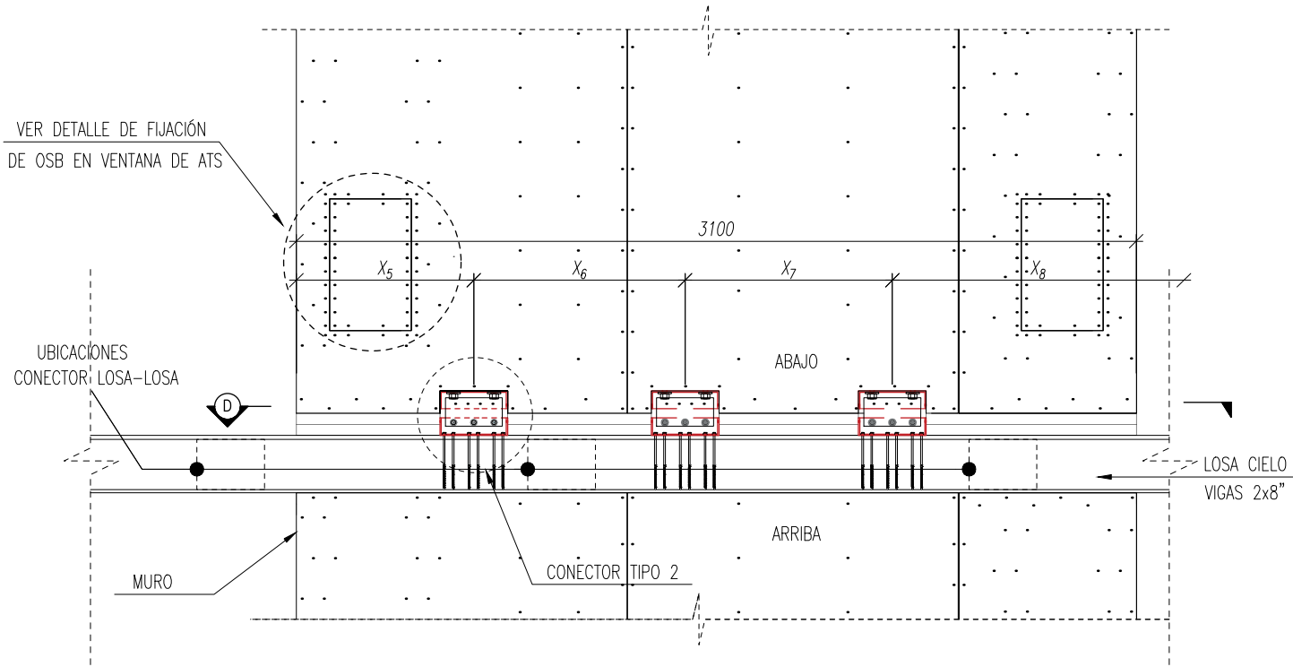
FIG. 14: DETALLE DE ACABADO O TERMINACIÓN DEL OSB EN VENTANA DE ATS PARA LOS MUROS DEL MÓDULO.
