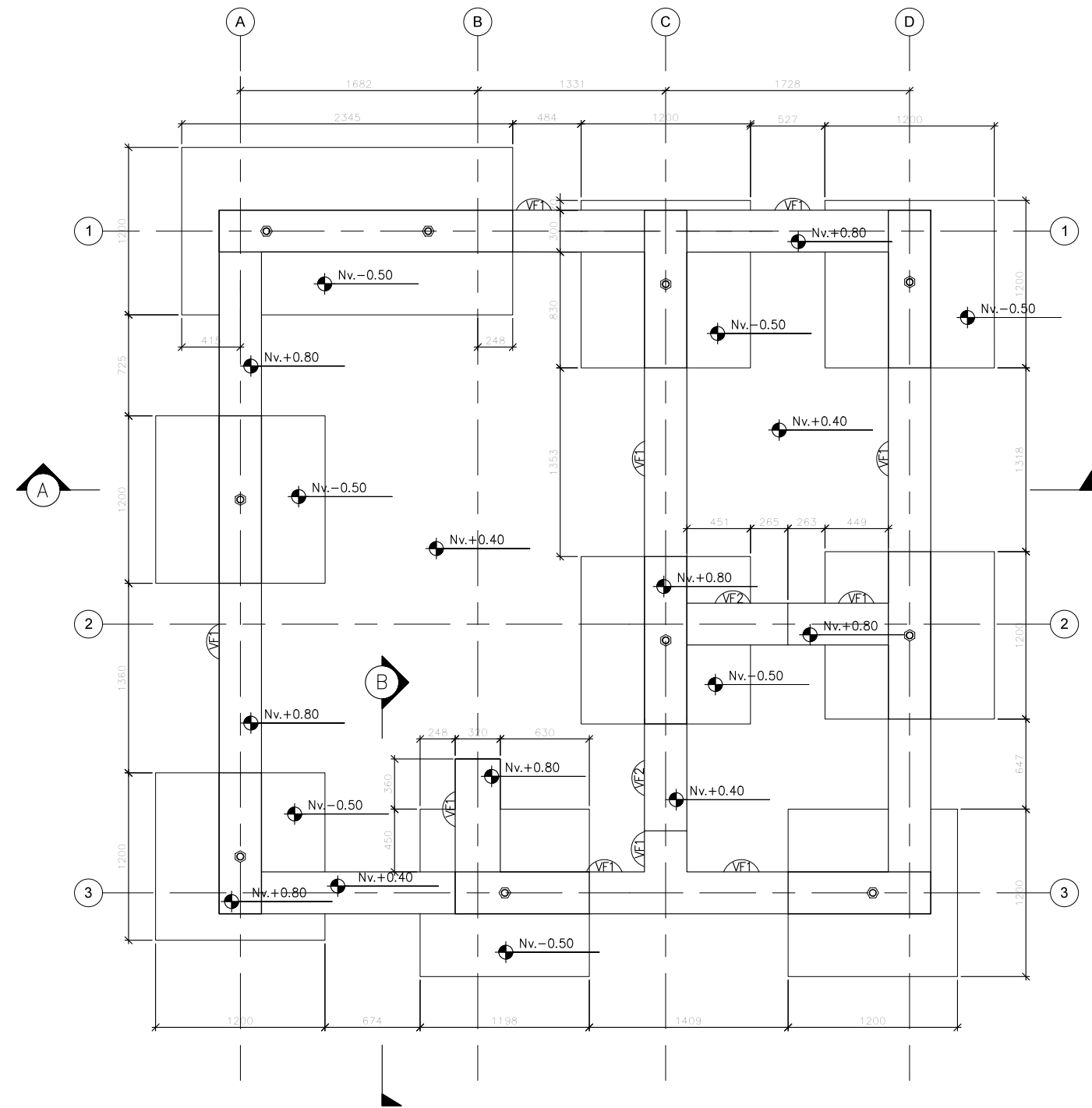
PLANTA DE FUNDACIONES ESCALA 1:25
