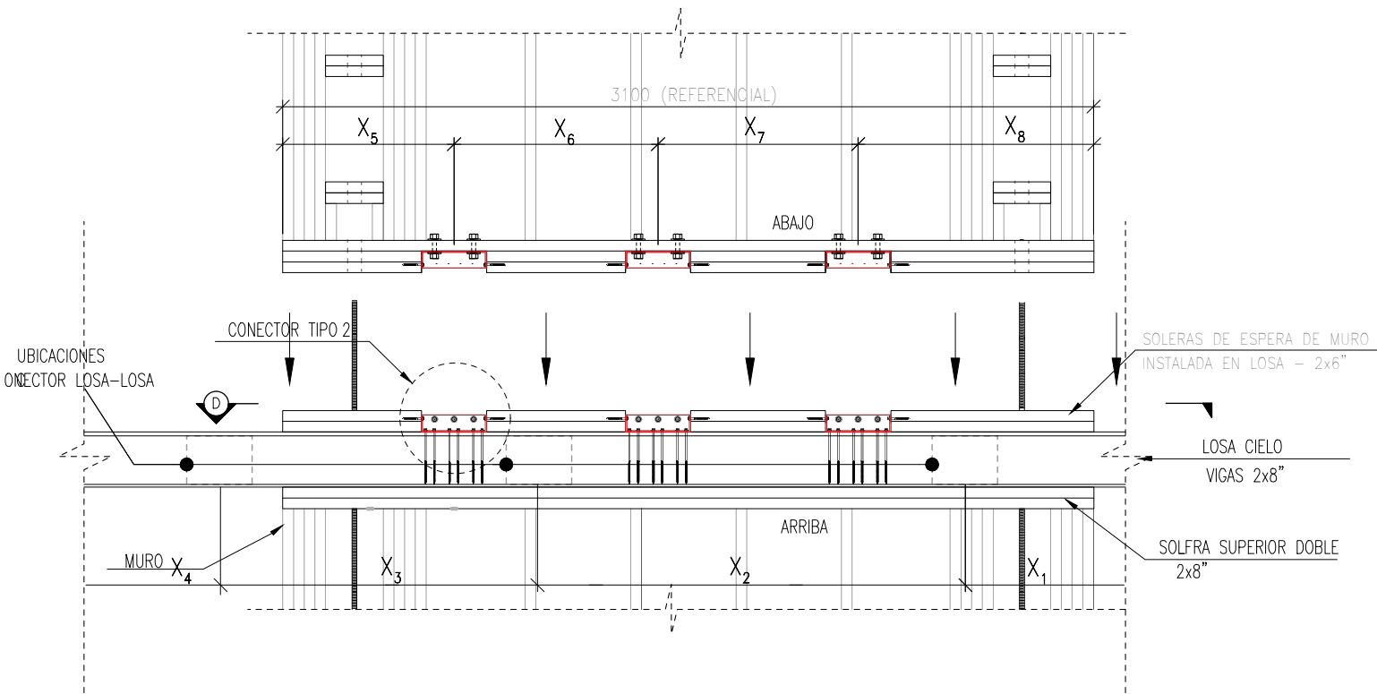
SECUENCIA PASO 1 VISTA EN ELEVACIÓN, CONEXIÓN MURO-LOSA DE UN PISO A OTRO
