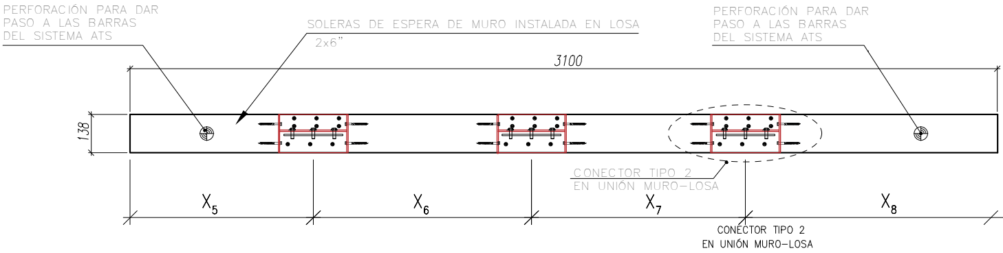
CORTE D-D
