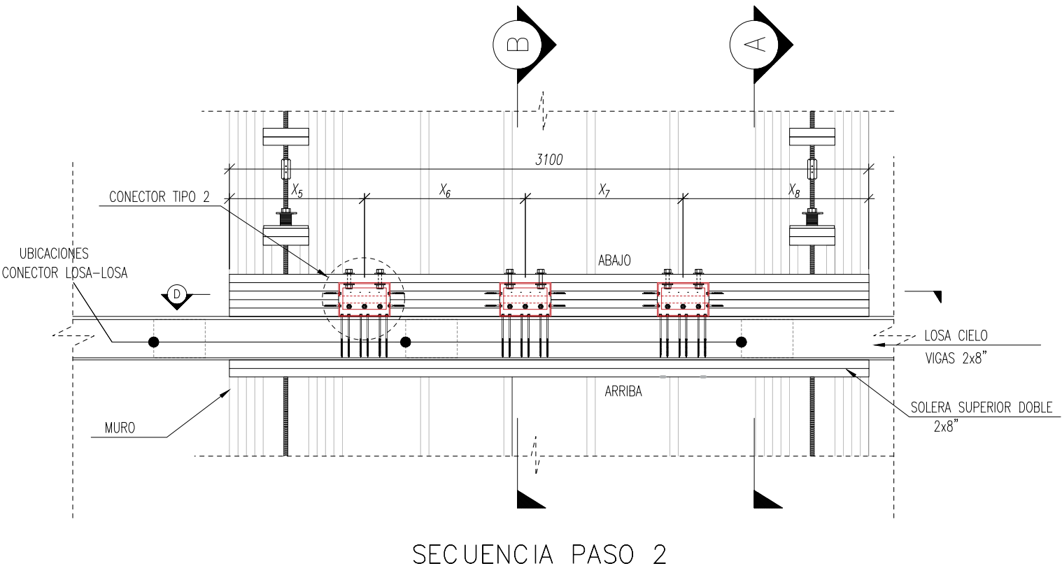
FIG.12: CORTE C-C, VISTA EN ELEVACIÓN DE CONEXIÓN MURO – LOSA (SIN TABLEROS DE REVESTIMIENTO)
