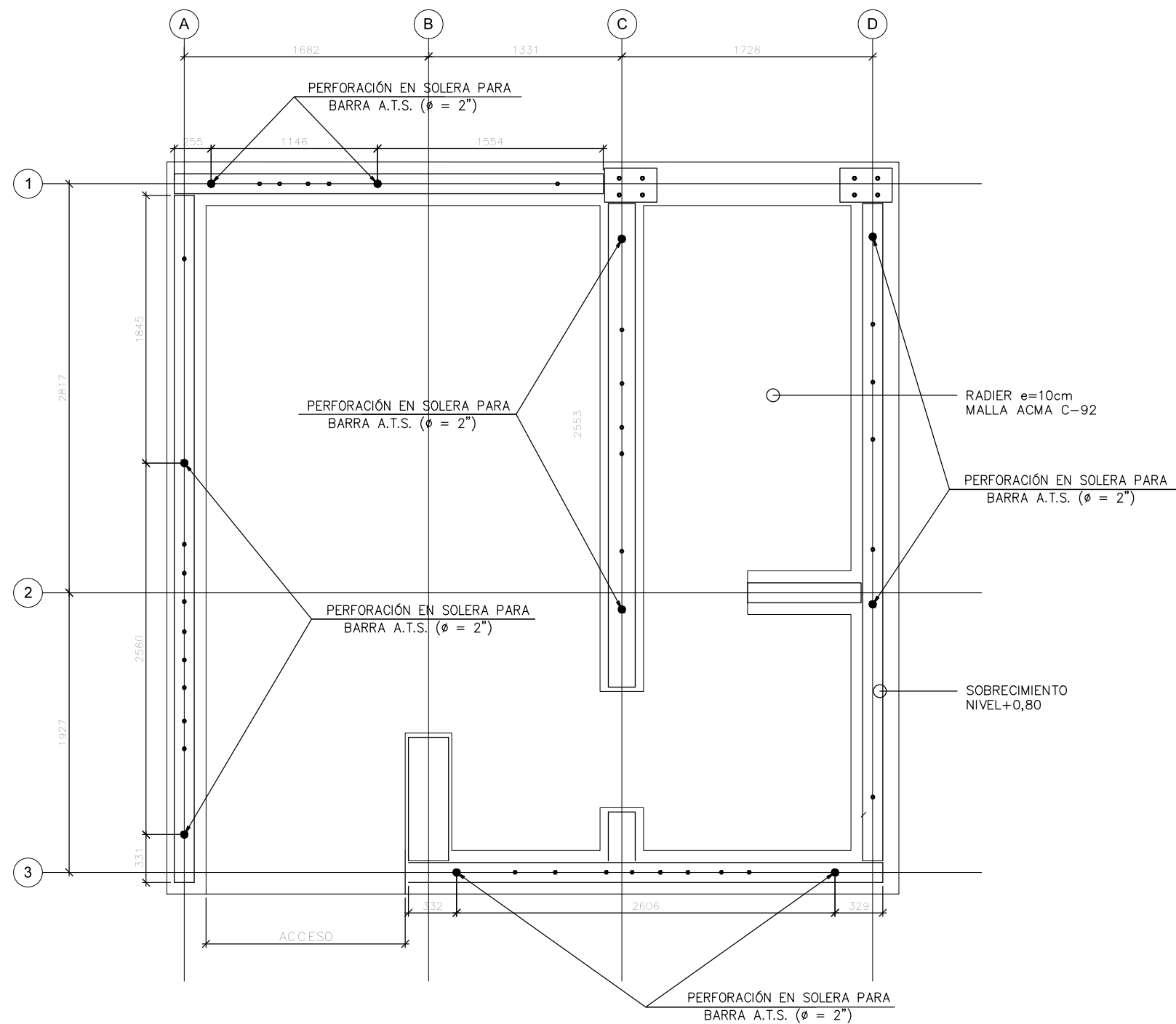
PLANTA DE SOLERAS DE ESPERA Y UBICACIÓN PERNOS DE ANCLAJE ESCALA 1:25
